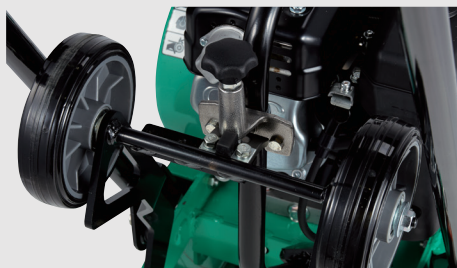
■ Butée pour chariot kit roues (MVC e-60 - MVC T60 - F80)
